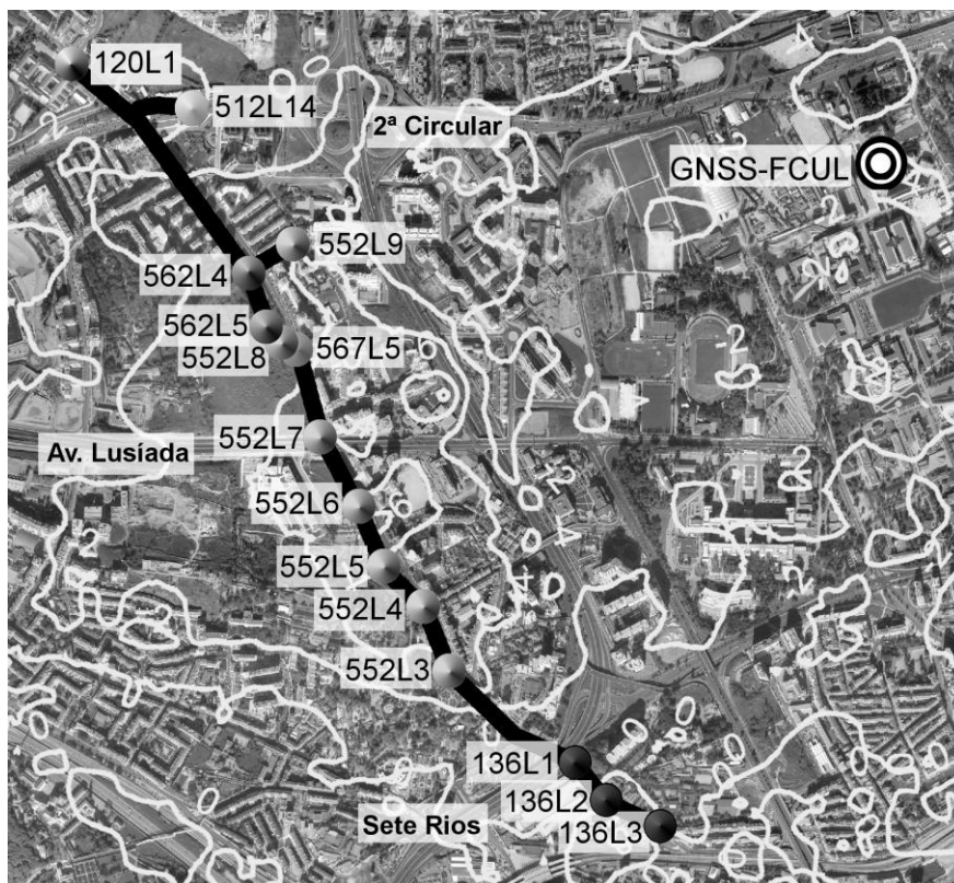
Figura 1 – Localização dos pontos nivelados nas estradas das Laranjeiras e da Luz. As isolinhas assinalam zonas de igual velocidade média de assentamento (mm/ano), de acordo com os dados PSINSAR
