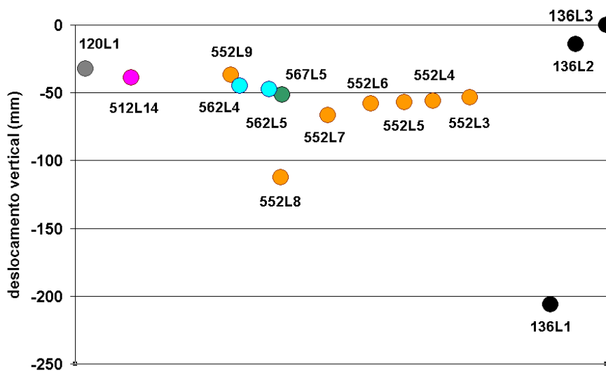
Figura 4 – Nivelamento geométrico: deslocamentos verticais entre 1995 e 2009
